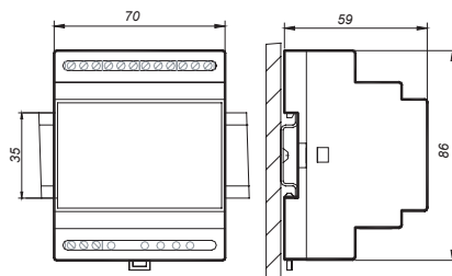
Габаритно-присоединительные размеры модуля ММ1
