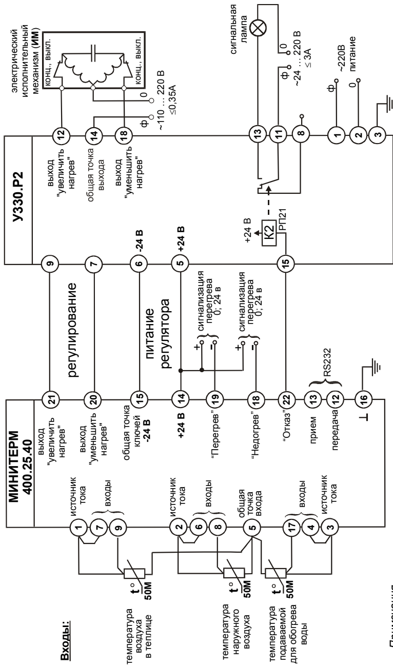
Рис. 3. Пример схемы подключения регулятора МИНИТЕРМ 400.25.40 в комплекте с усилителем УЗ30.Р2.
