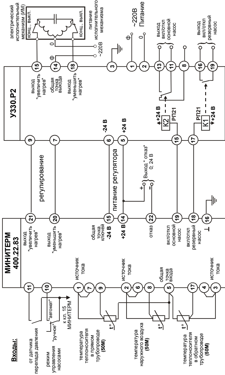
Рис. 1. Схема подключения регулятора МИНИТЕРМ 400.22.83 для регулирования температуры теплоносителя в системах отопления в комплекте с усилителем УЗ30.Р2
