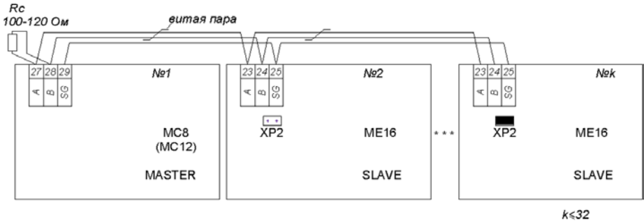
Рисунок 4 – Пример построения сети по интерфейсу RS485
