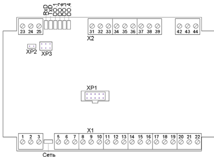
Рисунок 2- Плата модуля ME16
