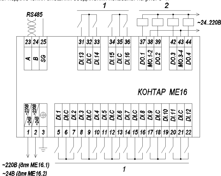
Рисунок 3 – Пример подключения внешних соединений к модулю ME16
