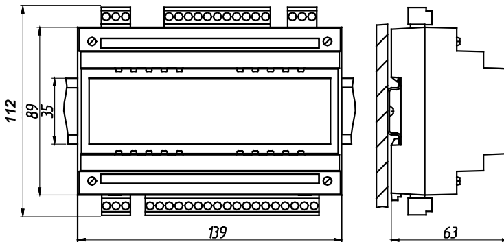
Рисунок 1 – Габаритно-присоединительные размеры модуля
